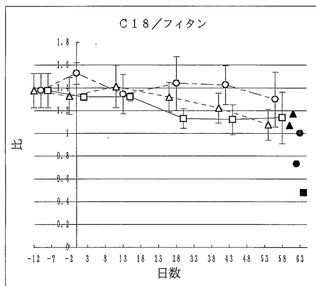
図6 油分解の経時変化状況
