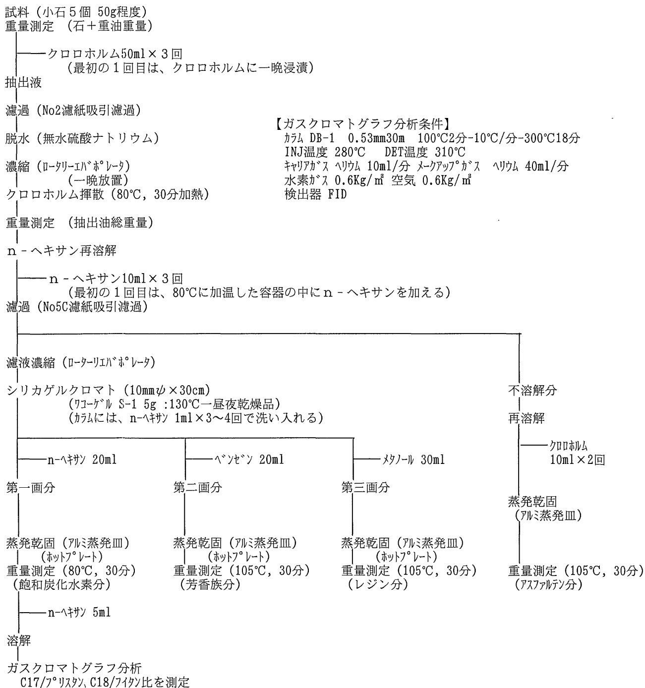
図 5 油成分分析のフローシート
