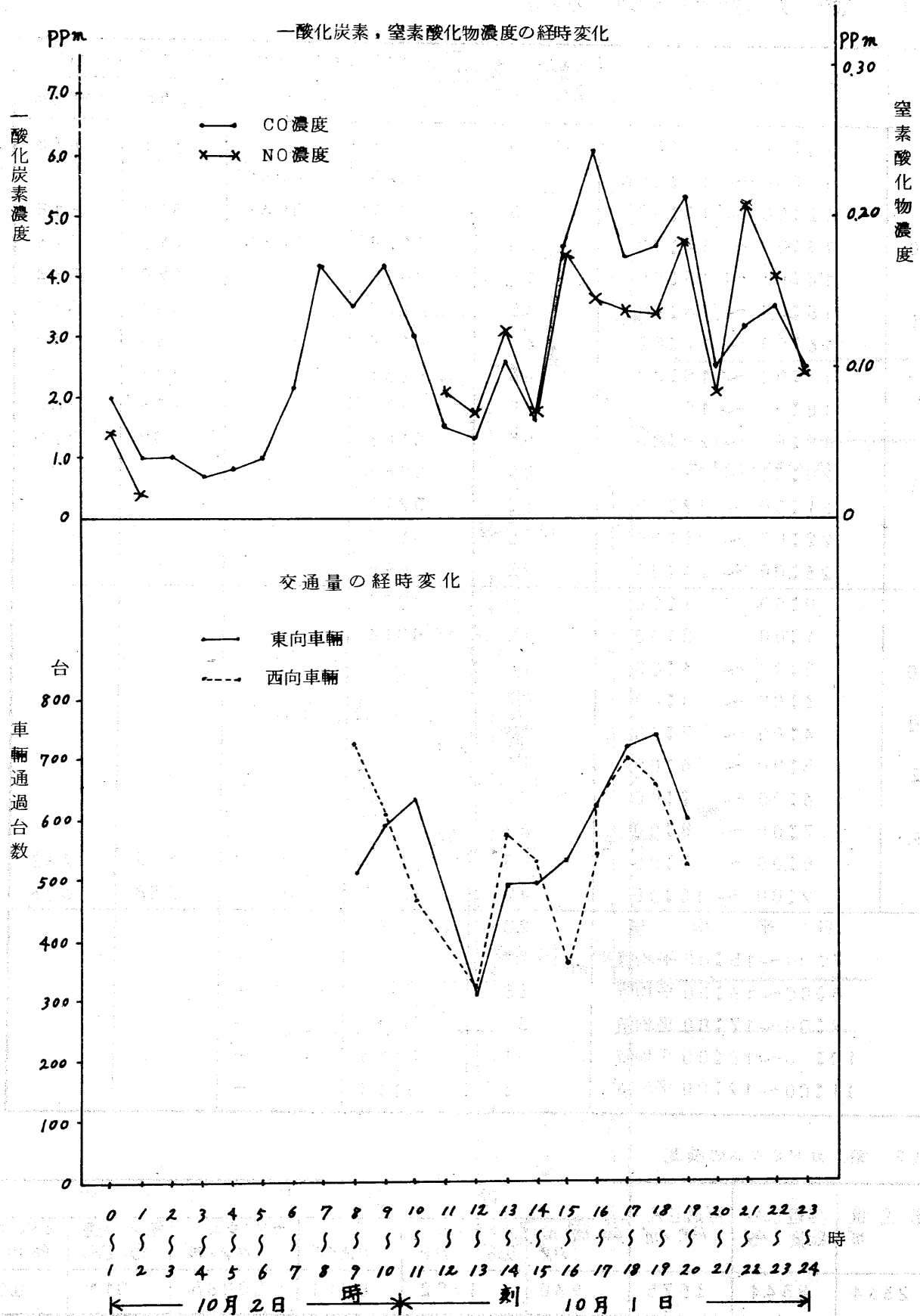
図2 一酸化炭素、窒素酸化物濃度と交通量
