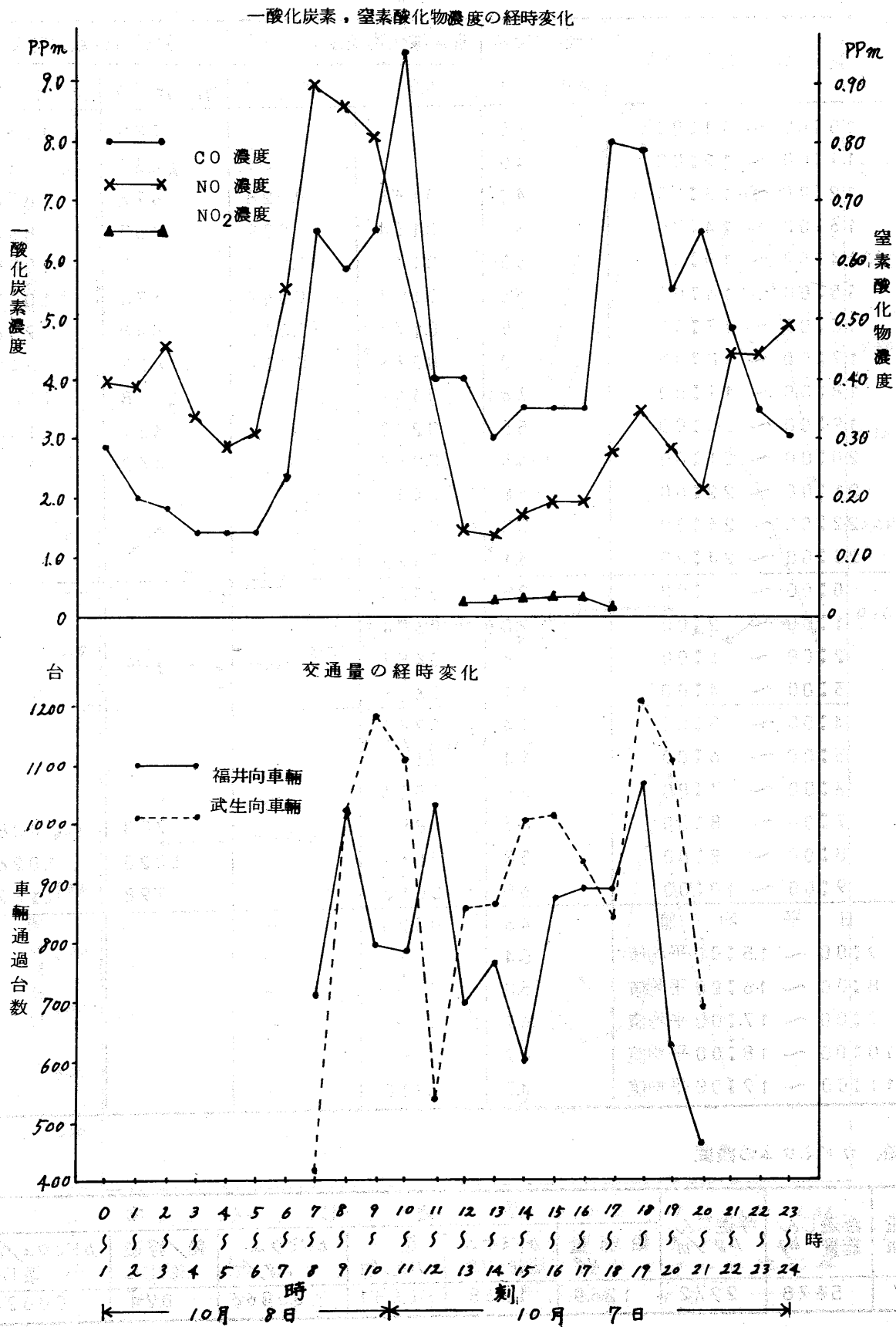
図4 一酸化炭素、窒素酸化物濃度と交通量
