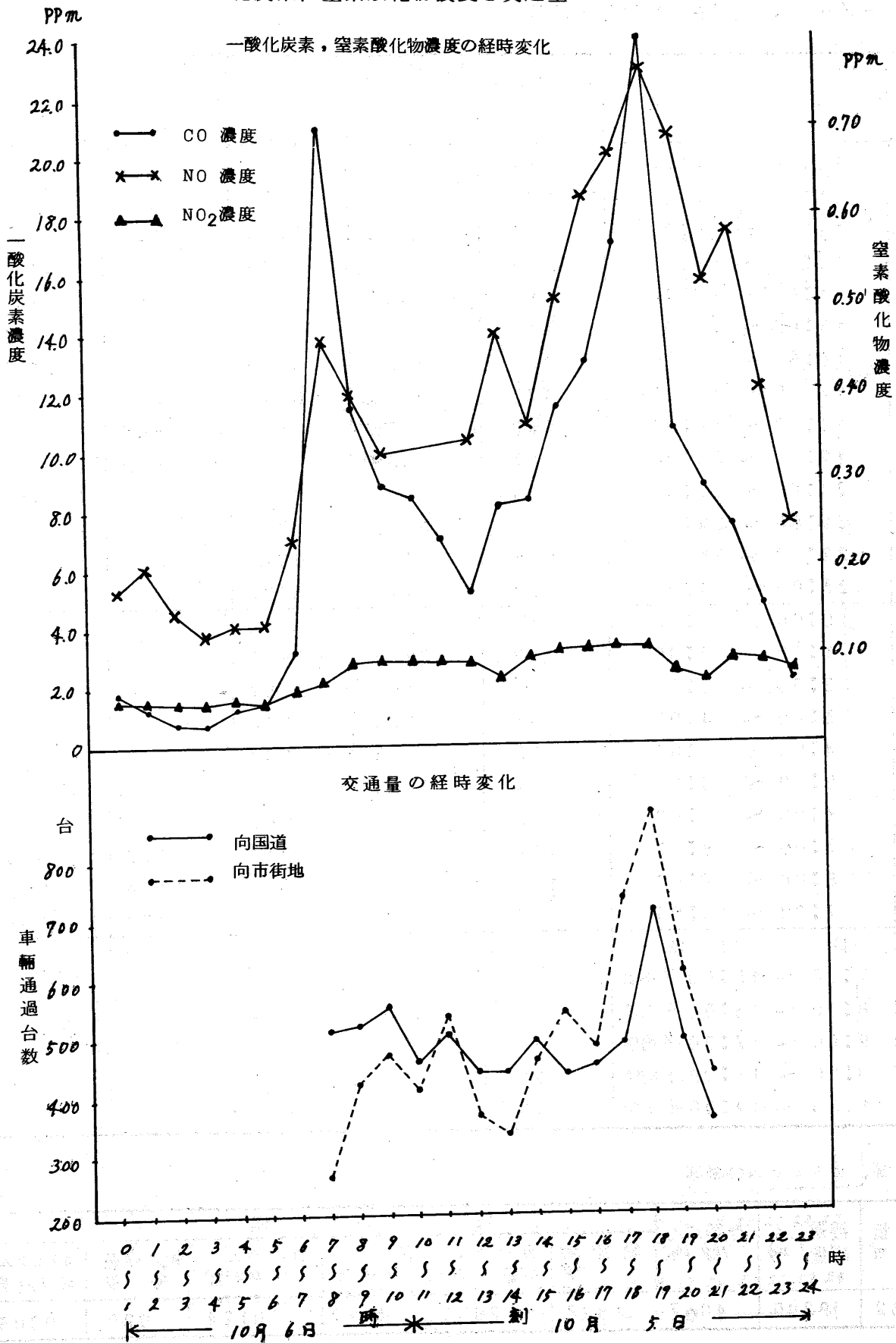
図3 一酸化炭素、窒素酸化物濃度と交通量
