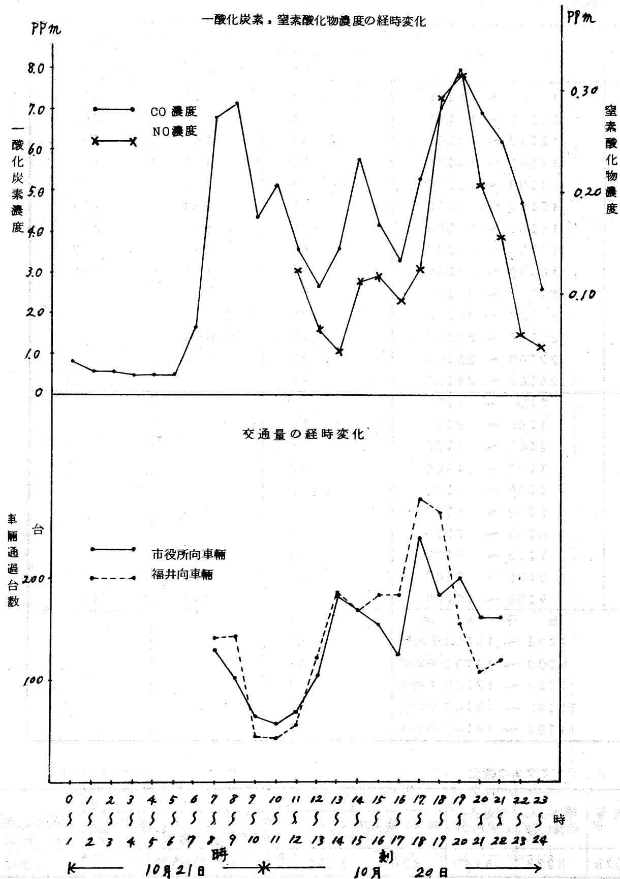
図6 一酸化炭素、窒素酸化物濃度と交通量
