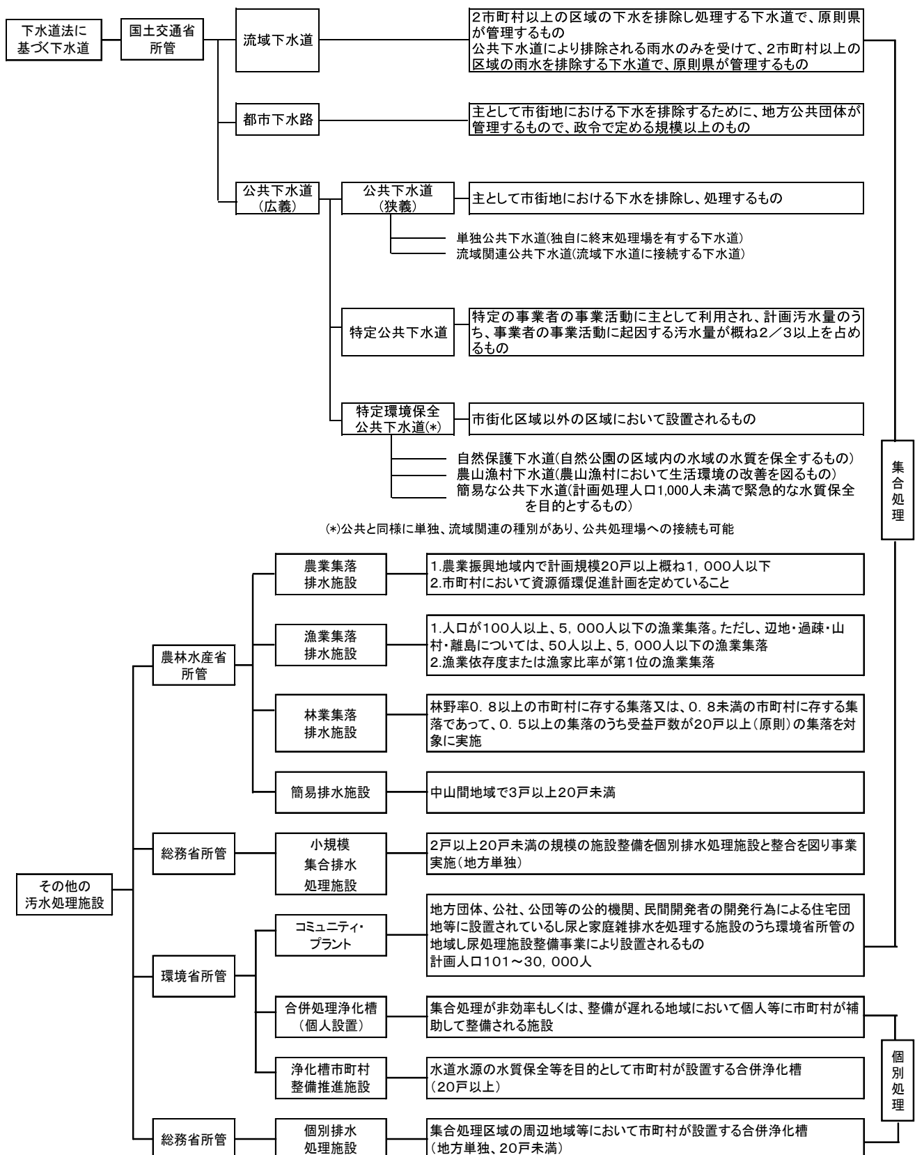
図4-1-13 污水处理施設の概要
