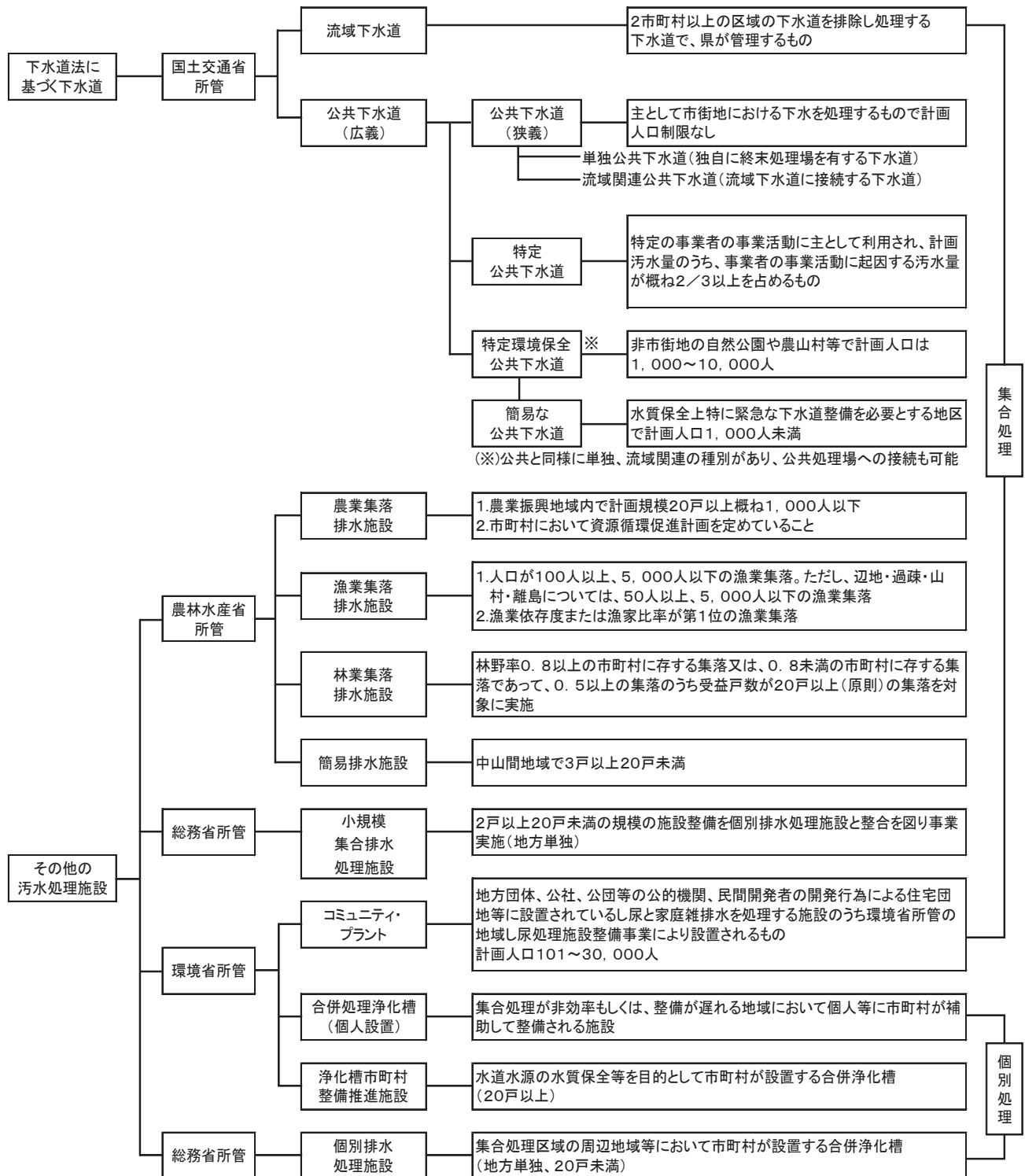
図4-1-13 污水处理施設の概要
