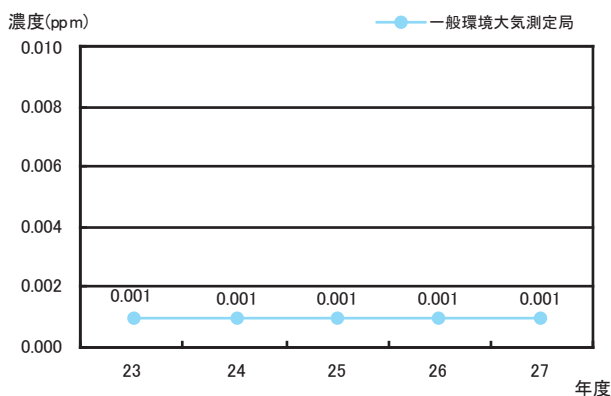
図4-1-28 二酸化硫黄の年平均値の推移
