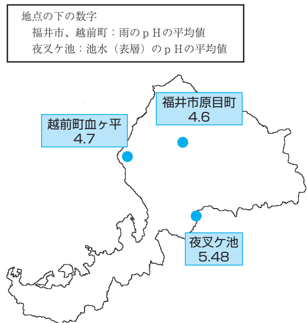
図4-1-48 酸性雨監視地点と平成27年度の監視結果
