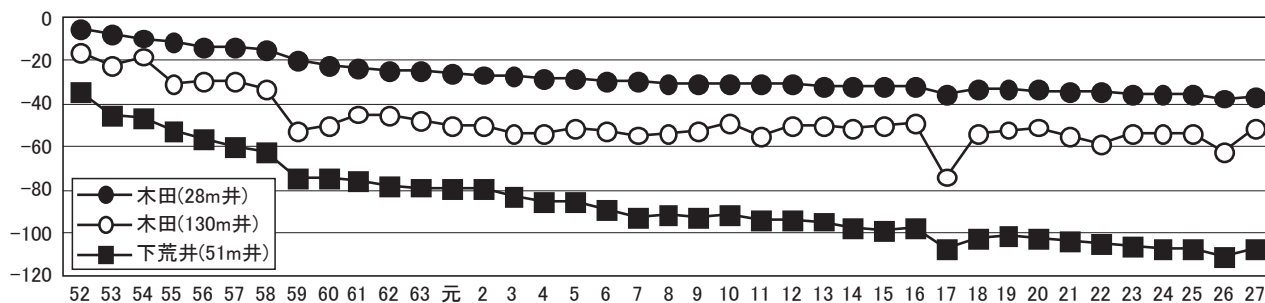
図4-1-24 福井市南部地域における地盤沈下の状況
