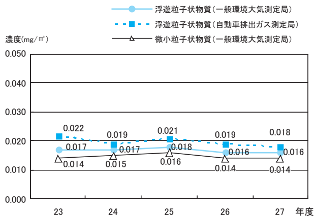
図4-1-30 浮遊粒子状物質・微小粒子状物質の年平均値の推移
