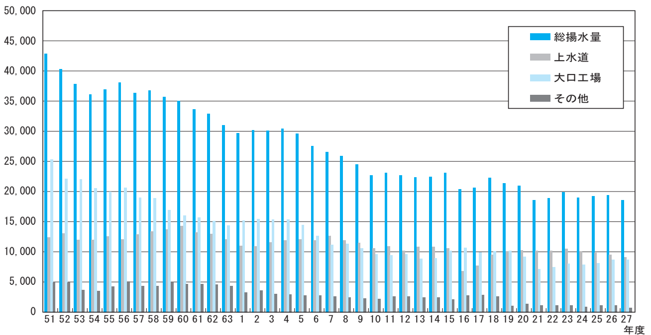
図4-1-25 福井市南部地域における地下水採取状況
