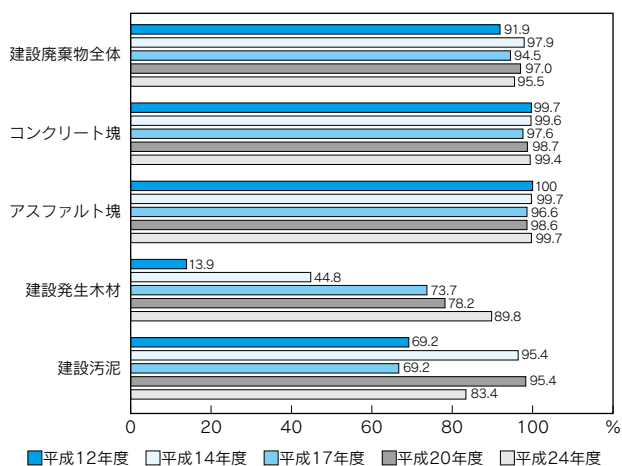
図3-1-15 建設廃棄物のリサイクル率
