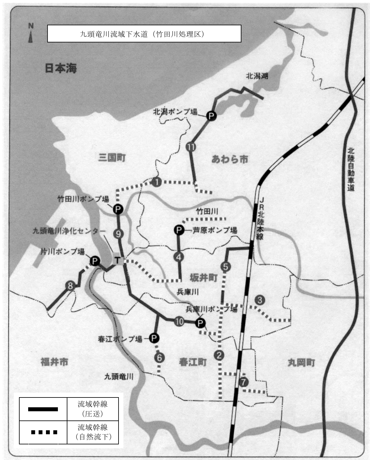
図 3-26 九頭竜川流域下水道計画図
