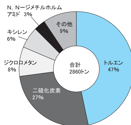
図3-3-76 大気への排出：物質別内訳
