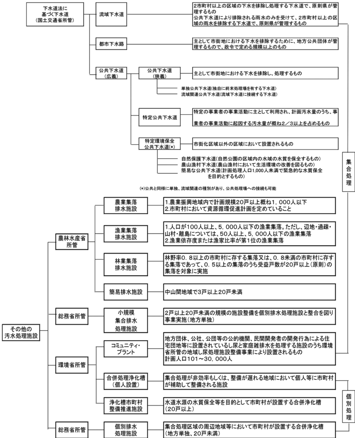
図 4-1-10 污水処理施設の概要
