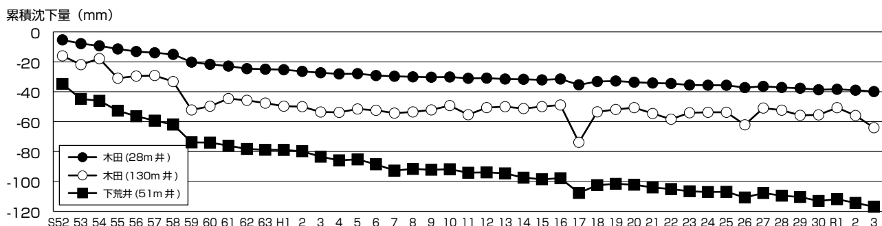
図 4-1-21 福井市南部地域における地盤沈下の状況
