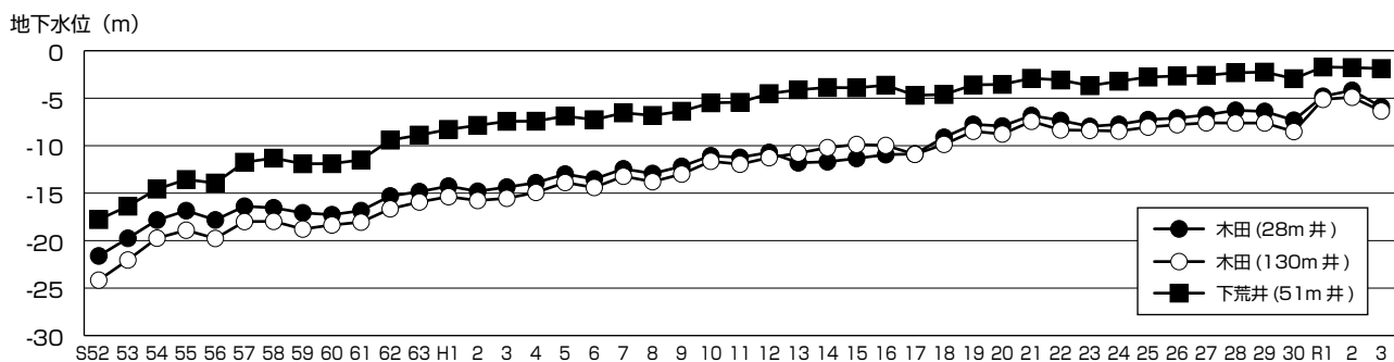
図 4-1-20 福井市南部地域における地下水位の状況
