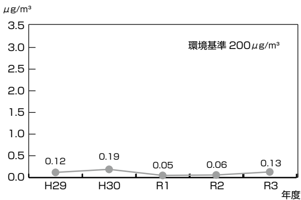
図4-1-35 テトラクロロエチレンの年平均値の推移
