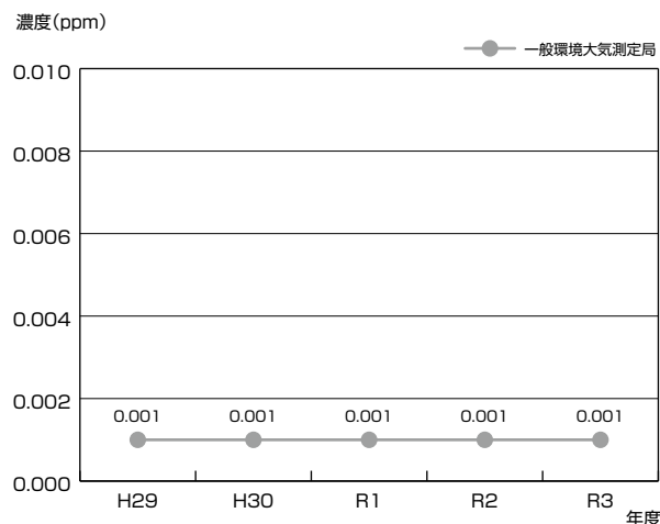
図4-1-25 二酸化硫黄の年平均値の推移
