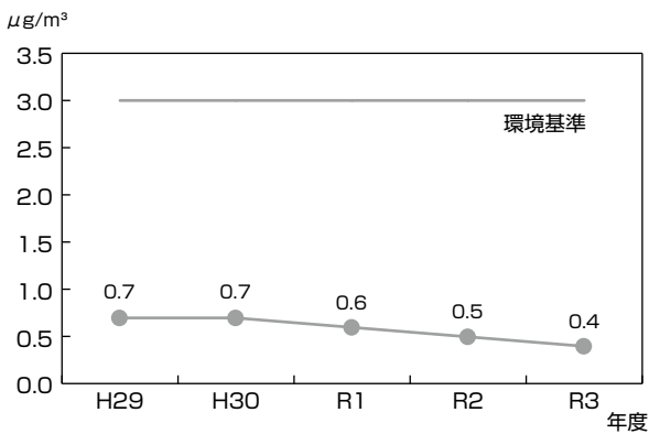
図4-1-33 ベンゼンの年平均値の推移
