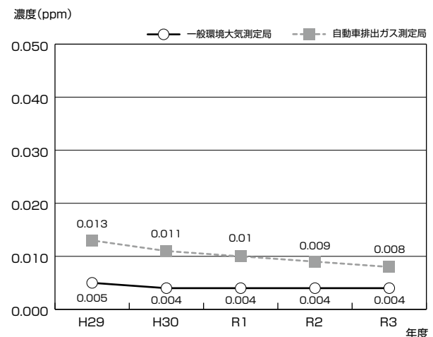
図4-1-26 二酸化窒素の年平均値の推移
