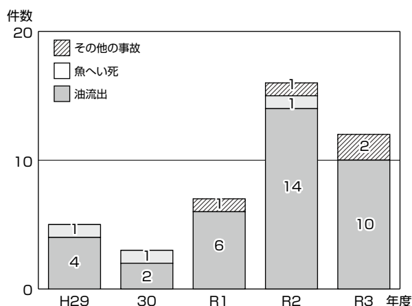
図4-1-51 水質事故発生状況の推移
