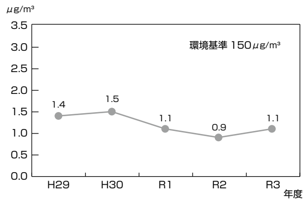
図4-1-36 ジクロロメタンの年平均値の推移
