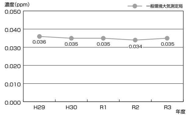
図4-1-29 光化学オキシダントの年平均値の推移
