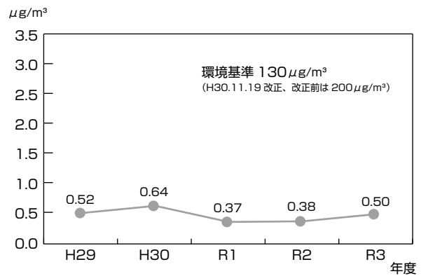
図4-1-34 トリクロロエチレンの年平均値の推移
