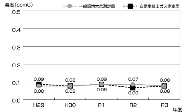
図4-1-30 非メタン炭化水素の年平均値の推移
