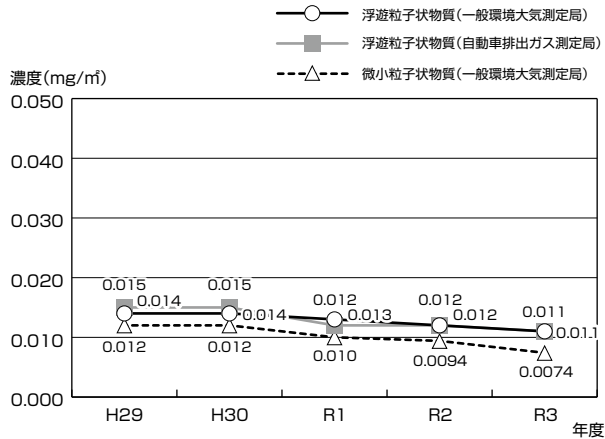
図4-1-27 浮遊粒子状物質・微小粒子状物質の年平均値の推移
